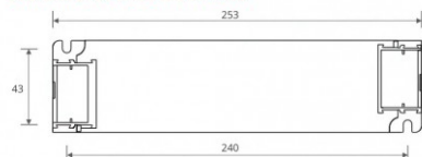
Dimensions en mm de face sans les caches
