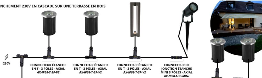
BRANCHEMENT 230V EN CASCADE SUR UNE TERRASSE EN BOIS
