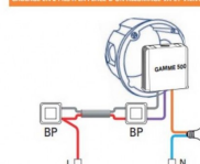
CÂBLAGE EN 2 FILS À LA PLACE D'UN ALLUMAGE VA-ET-VIENT
