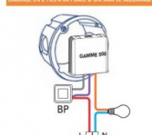
RECOMMANDATION DE LA PUISSANCE SUR UN CIRCUIT AVEC LA SÉRIE 500
