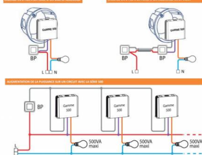
CÂBLAGE D'UN TÉLÉRUPTEUR MTV500E
