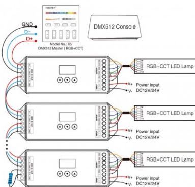
Diagramme de connexion
