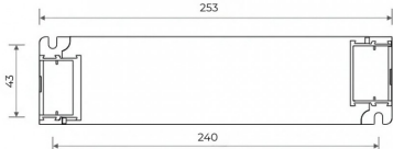
Dimensions en mm de profil
