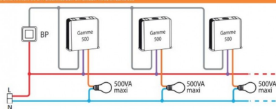
RECOMMANDATION DE LA PUISSANCE SUR UN CIRCUIT AVEC LA SÉRIE 500
