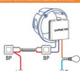
CÂBLAGE EN 2 FILS À LA PLACE D'UN ALLUMAGE VA-ET-VIENT
