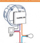
RECOMMANDATION DE LA PUISSANCE SUR UN CIRCUIT AVEC LA SÉRIE 500
